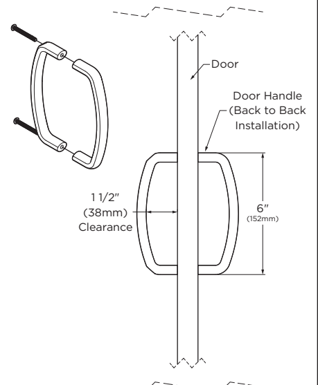
#1000312 Door Pull Handle
