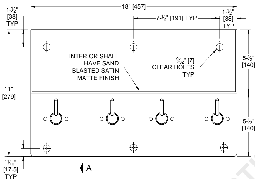
ELEVATION
